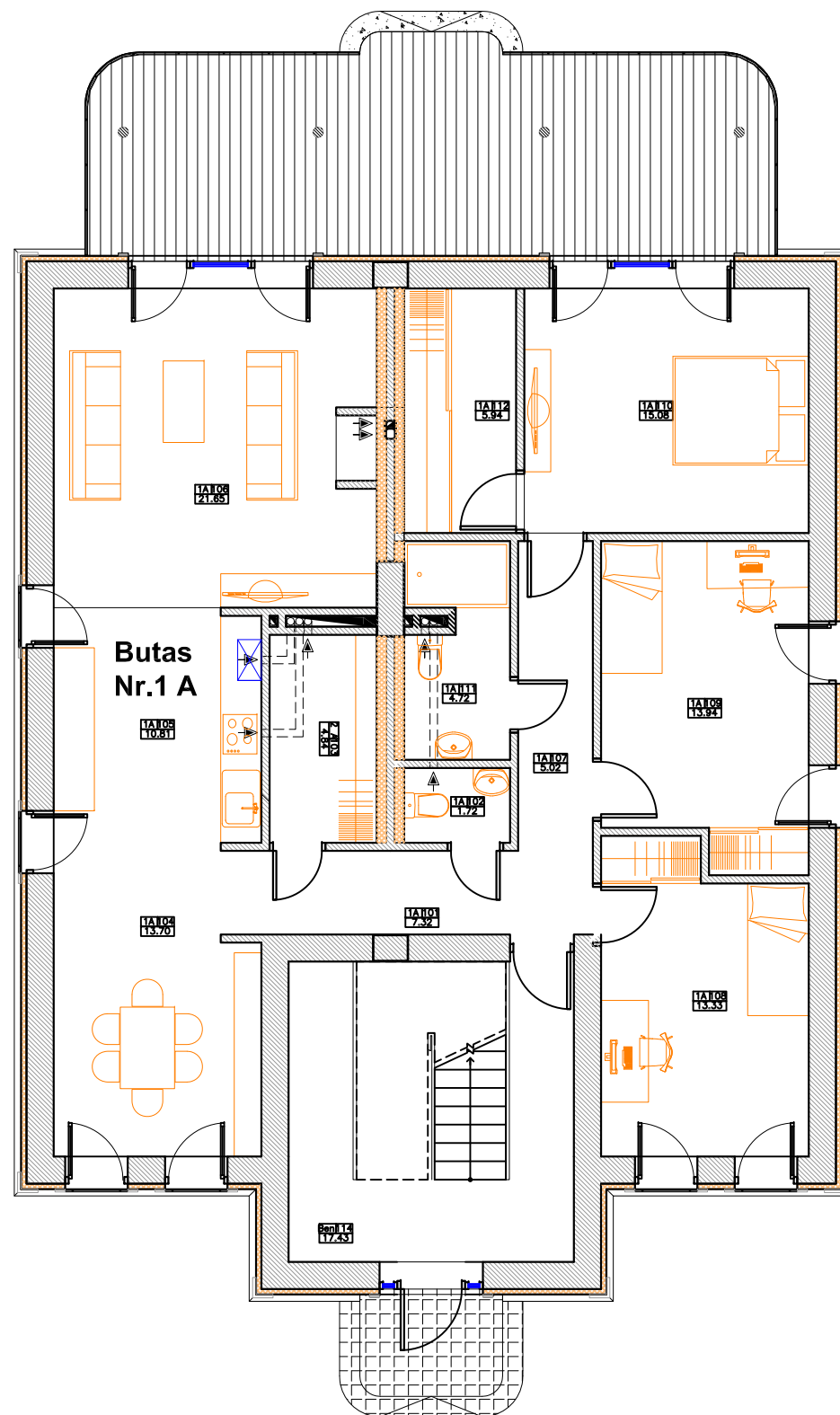
I aukšto patalpų eksplikacija
